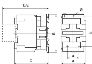
CJX2-D40-95
